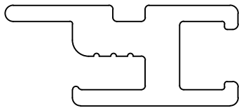
DETAIL A-A SCALE 2:1
